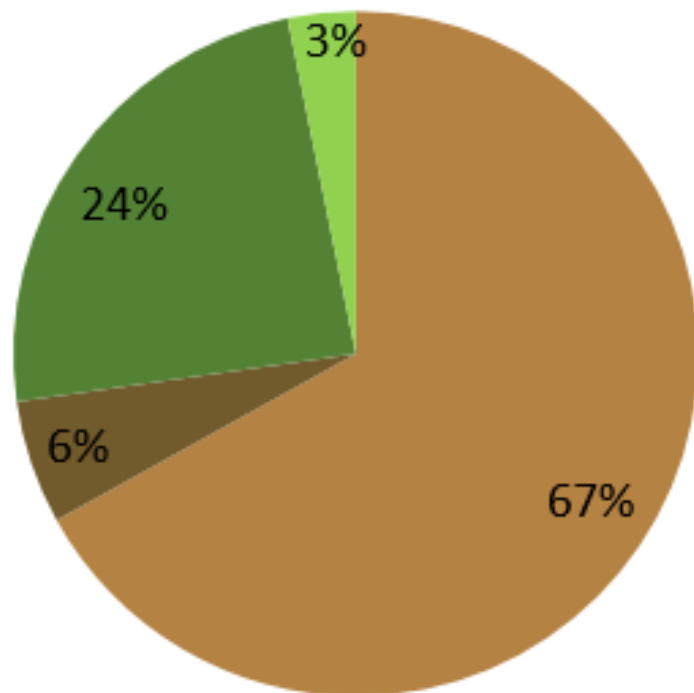
Hainbuche Trockenmasse
