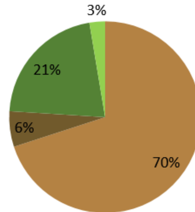
Ahorn Trockenmasse
